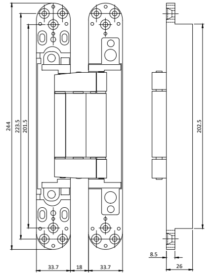
CUTOUT DIMENSIONS
