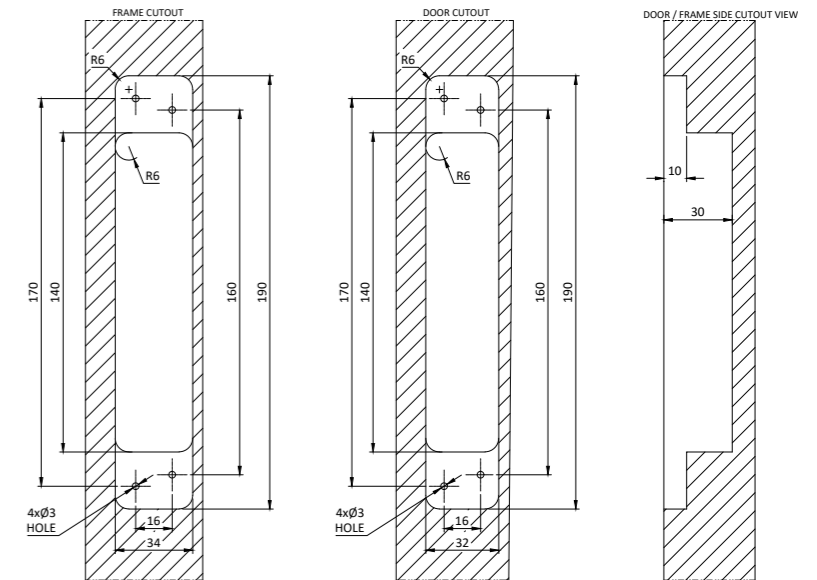
CUTOUT DIMENSIONS
