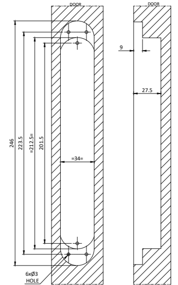
CUTOUT DIMENSIONS
